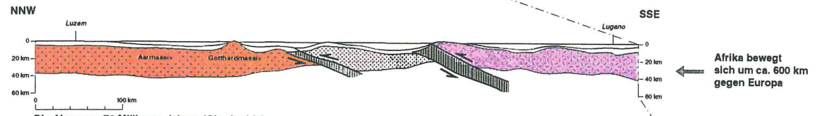
Die Alpen vor 70 Millionen Jahren (Oberkreide)
