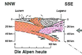
Die Alpen heute
