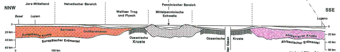
Die Alpen vor 110 Millionen Jahren (Unterkreide)
