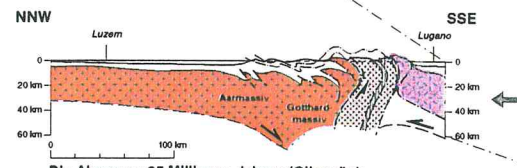
Die Alpen vor 35 Millionen Jahren (Oligozän)
